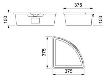
Art. OM 4.0504 RUOTE / WHEELS Possibilità di 4 ruote diametro 4 cm Altezza totale (con ruote) 34 cm. Possibility 4 wheels 4 cm diameter, total size 34 cm.
