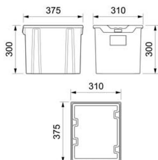
Art. OM 4.0498 VASCHETTA H. 30 TRAY H. 30 polipropilene / polypropilene Dim. cm. 37,5 x 31 x 30 h
